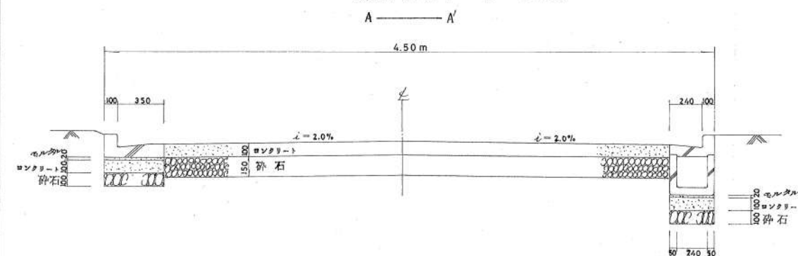
道路横断面 S = 1:20
