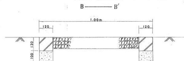
道路横断面 S = 1:10
